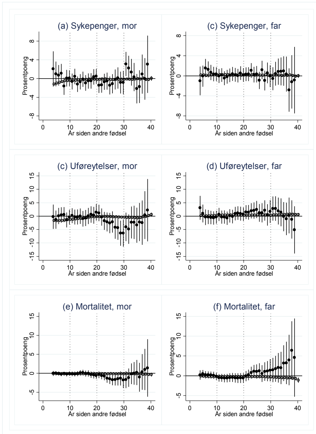
Figur 4. Årlige estimater av effekten av antall barn på sykefravær, uførehet og mortalitet
